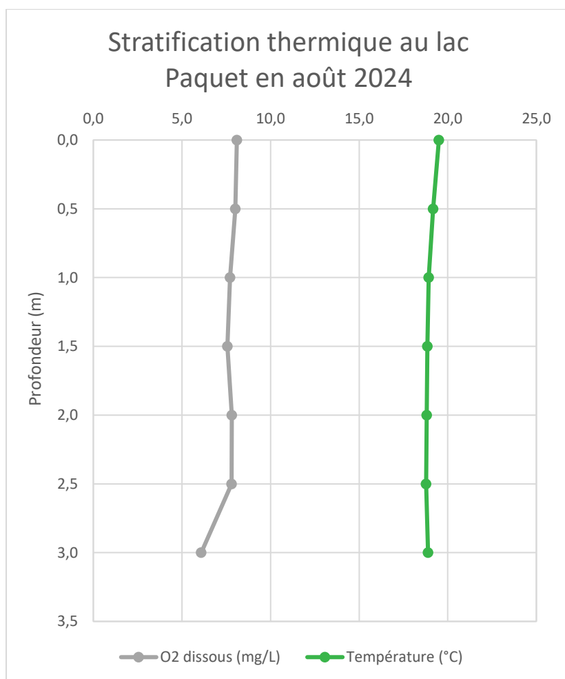
FIGURE 1 : RÉSULTAT DU PROFIL DE TEMPÉRATURE ET D'OXYGÈNE DISSOUS IN SITU EFFECTUÉ LE 3 SEPTEMBRE 2024 AU LAC PAQUET
